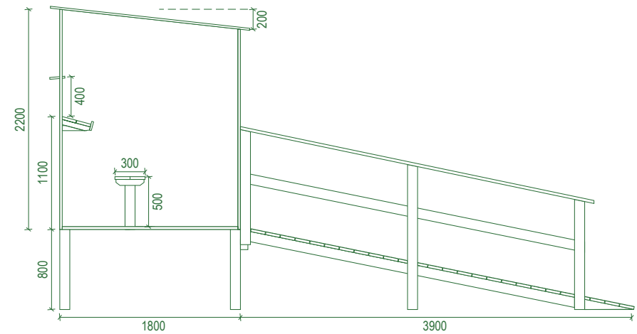
VUE LATÉRALE
